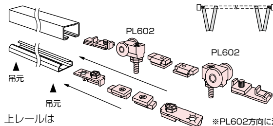
図B レール部品の差し込み順序と方向 (吊ガイド式WCB部品セット例)
