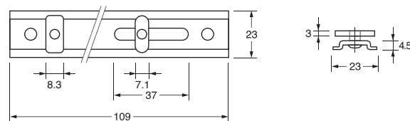
W1M 角座(巾 8.3) W1S R座(巾 7.1)
