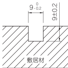
● 敷居材掘込み寸法
