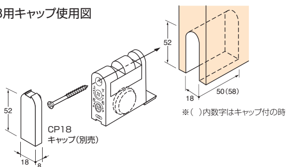
25-2D-18用スペーサー使用図
