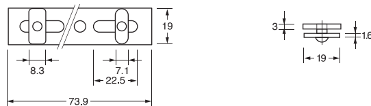
S1M 角座(巾 8.3) S1S R座(巾 7.1)
